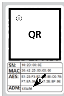
QR-Code Aufkleber Motorschloss
